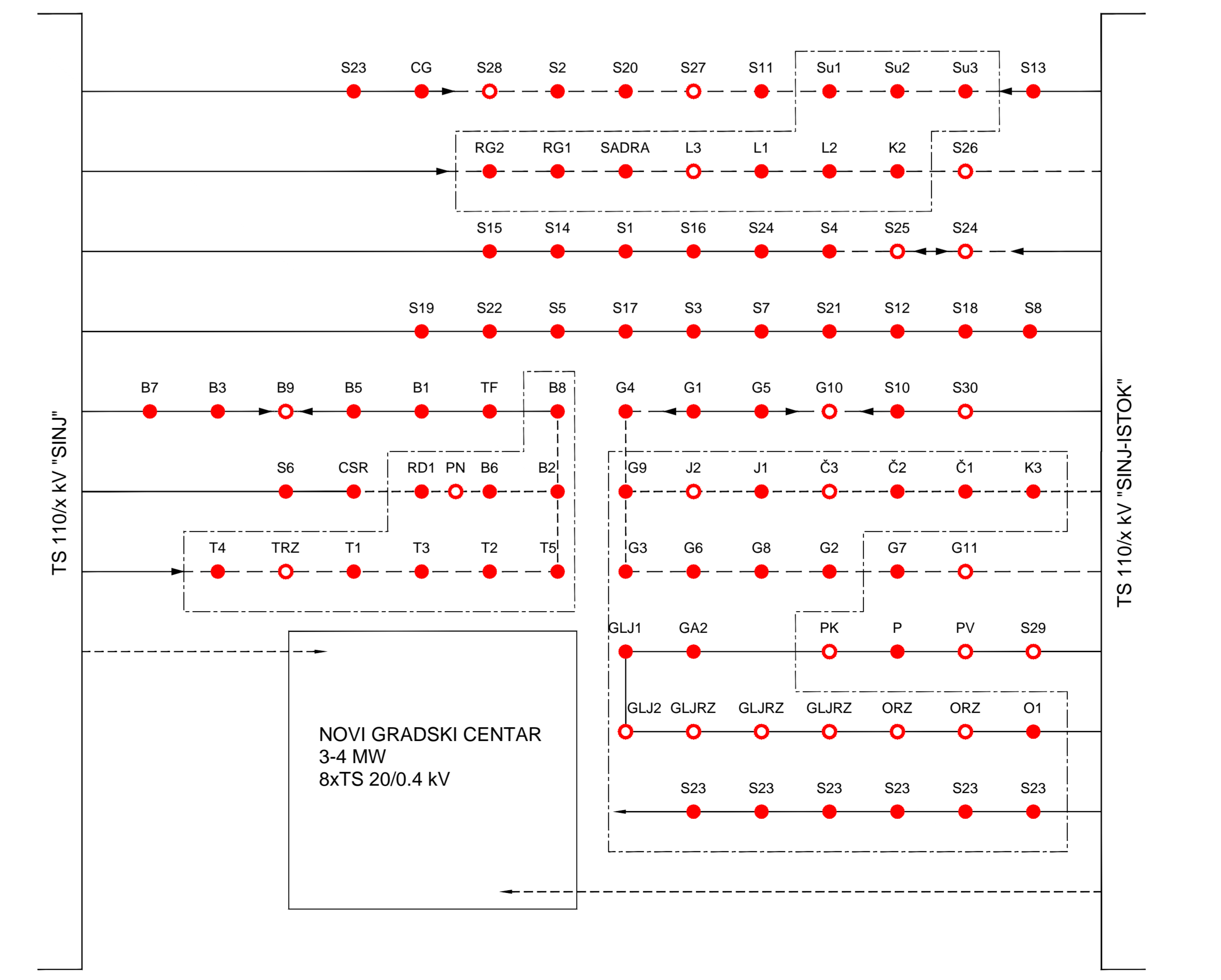
JEDNOPOLNA SCHEMA PERSPEKTIVNE ELEKTRIČNE MREŽE 20(10)kV GRADA SINJA
